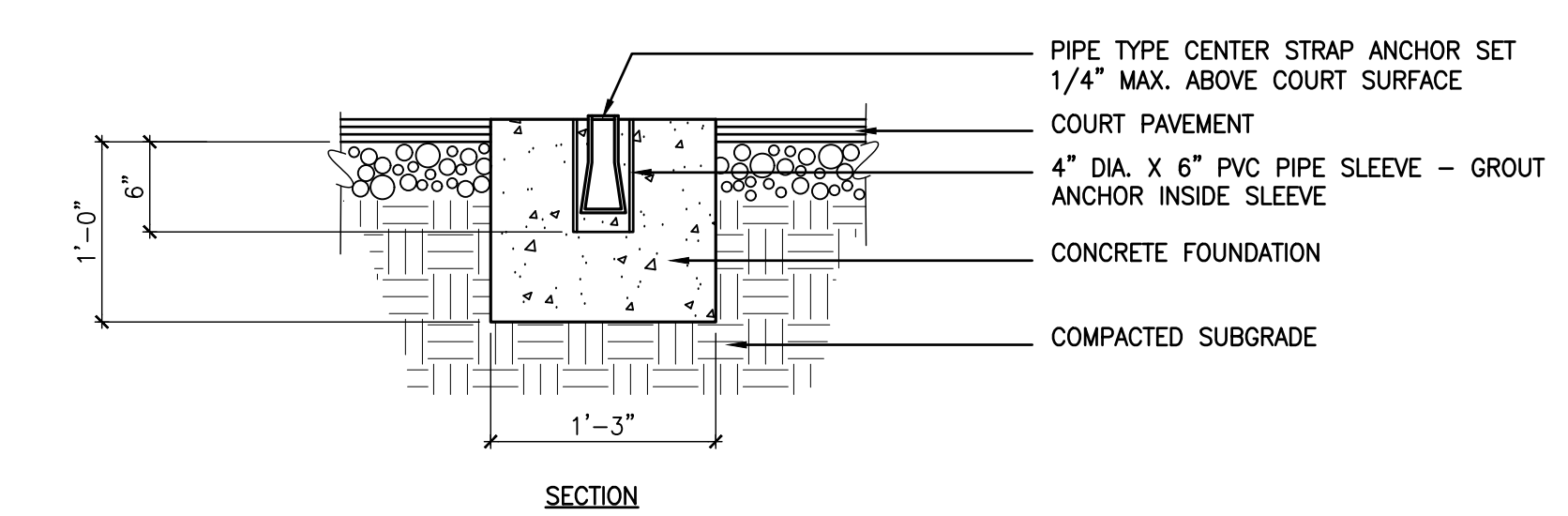
3 CENTER STRAP ANCHOR DETAIL SCALE: 1"=1'-0"
